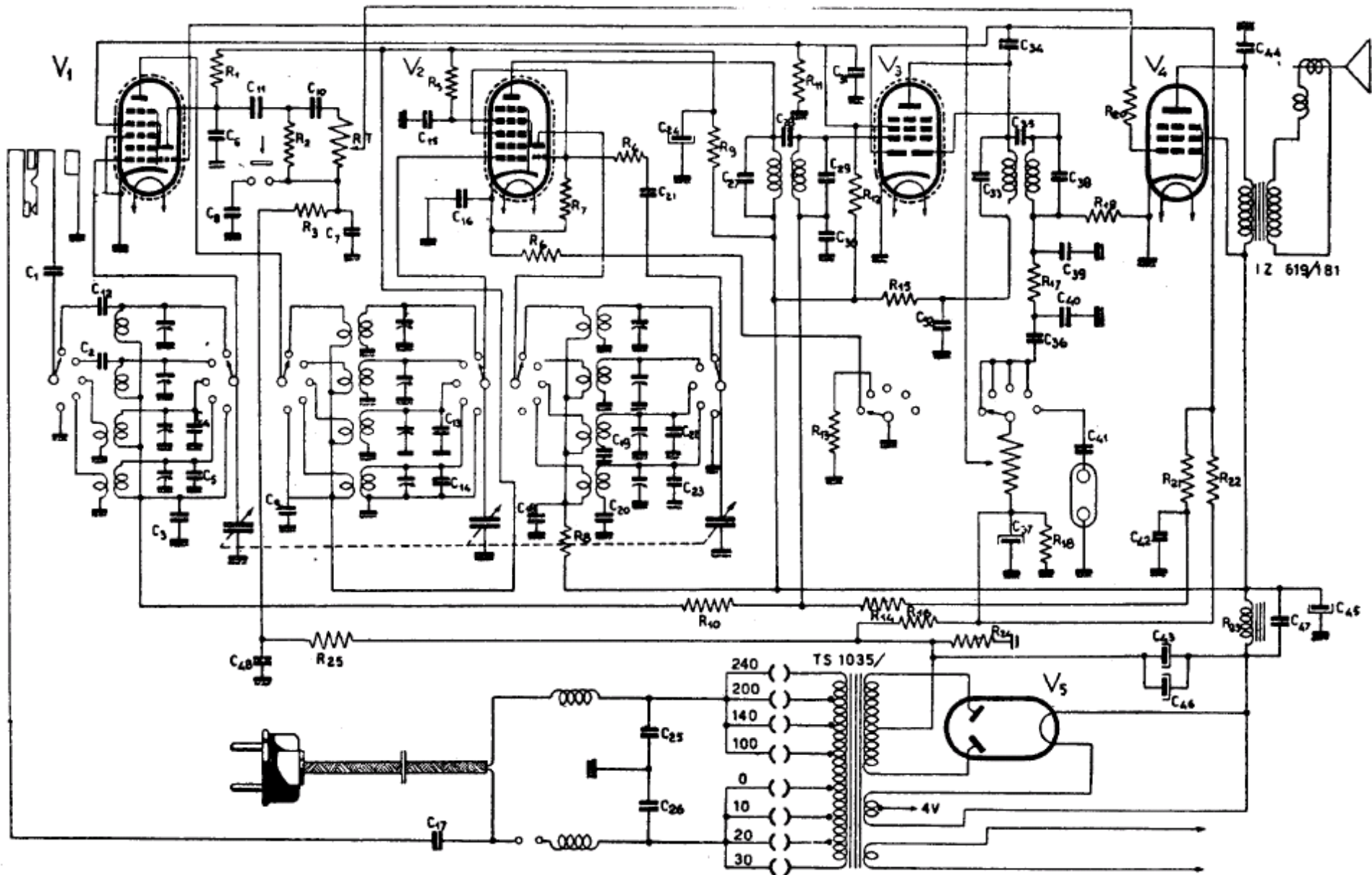
PHONOLA RADIO - Mod. 571 - Quattro gamme di ricezione. Media frequenza: 470 kc/s. Prima ECH4 amplificatrice AF e BF, seconda ECH4 convertitrice. V3-EBF2 o WE19. V4-EL3. V5-5Y3 G o WE54. Produzione 1946.
